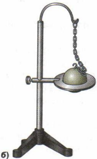
Рис. 18. Тепловое расширение металлического шара
